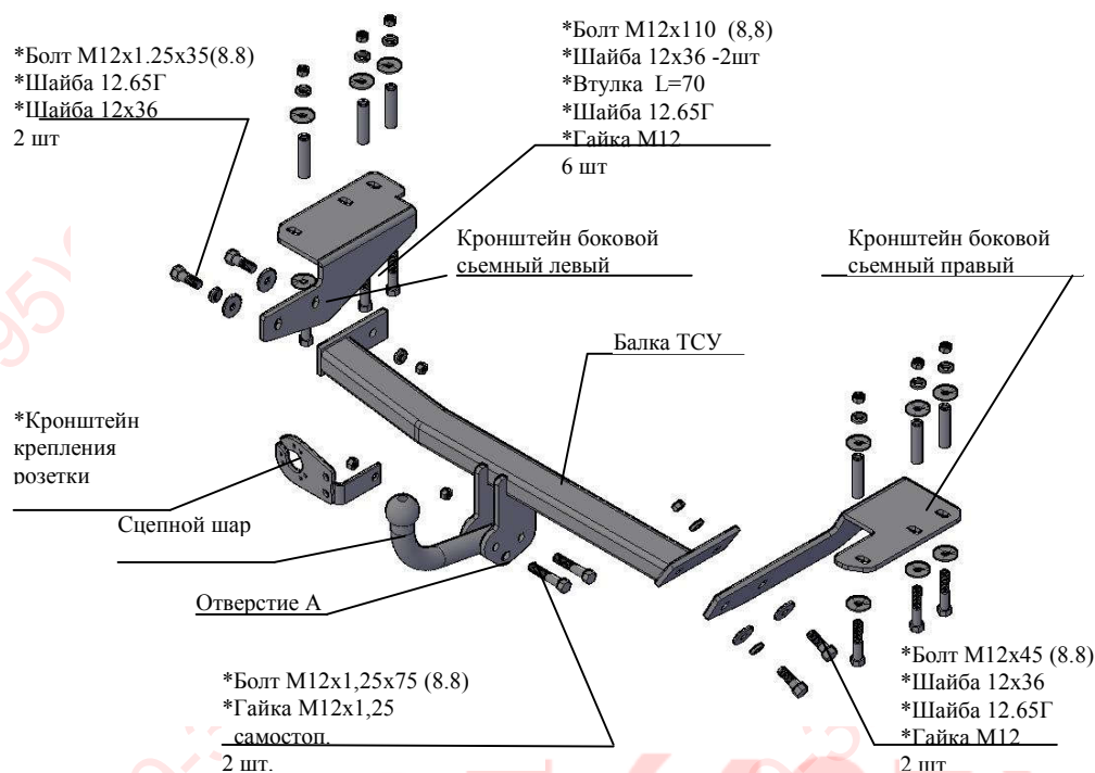
Рис.1 Тягово-сцепное устройство 8121.
